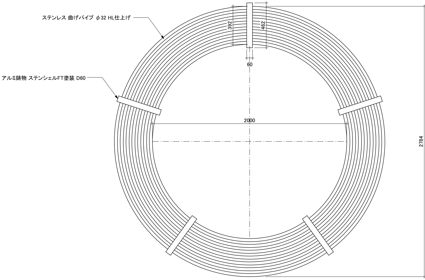
平面図
