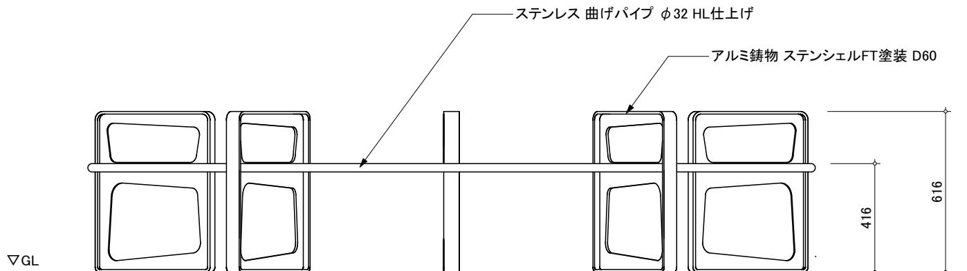
正面図
