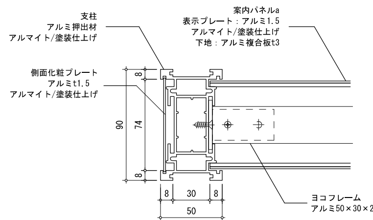
断面図S=1/3
