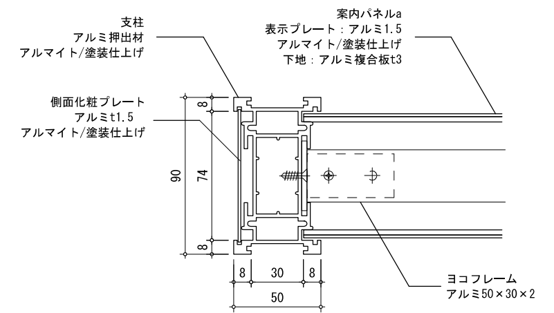
断面図S=1/3
